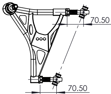
MAX LENGTH
